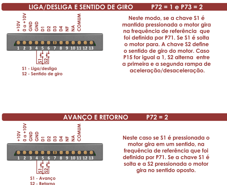
Figura 9-2 - Opções de comando através dos bornes de controle
