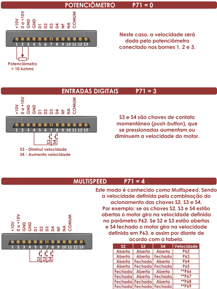
Figura 9-1 - Opções de referência de frequência (velocidade) através dos bornes de controle
